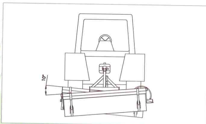
Pendelausgleich im Dreipunkturm
