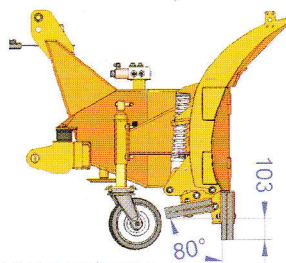
Bild 1 Federsicherung
