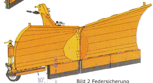
Bild 2 Federsicherung
